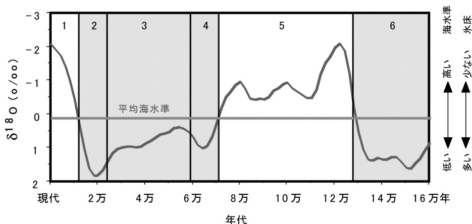
第1図 過去16万年における海水の酸素同位体比変動。Y軸は通常と逆にプロットしてある。上側は氷床量が少ないので海面が高く、下側は逆に氷床量が多いので海面が低いことを表す。酸素同位体比 ^{18}\text{O}/^{16}\text{O} は、 \delta^{18}\text{O} = ((^{18}\text{O}/^{16}\text{O})_{\text{試料}} / (^{18}\text{O}/^{16}\text{O})_{\text{標準物質}} - 1) \times 1000 より、標準物質との千分偏差として定義される(単位:パーミル)。世界標準物質であるPDB (Peedee層産ベレムナイト化石)が枯渇してしまったため、現在は、石灰岩試料であるNBS-19 ( \delta^{18}\text{O} = -2.20 パーミル)を用いて標準化される(VPDBスケール)。第四紀の氷期・間氷期の研究では、よりわかりやすくするために、期間ごとにステージ番号が付けられている。すなわち、偶数番号が氷期、奇数番号が間氷期が原則であり、図中で氷期は灰色で表示されている。例外的にステージ3のみは、ステージ2, 4より氷床の発達が改善されたが、実際には氷期の特徴をより強く示すので灰色で表示した。なお、最終氷期最盛期は2万5,000年～1万8,000年前の間とする人もいる(IPCC, 2001)。
