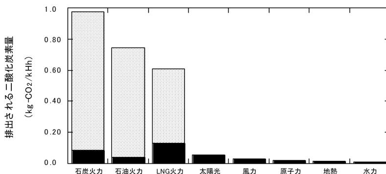
第8図 日本の電源別ライフサイクルアセスメント二酸化炭素の比較(電機事業連合会, 2005)。暗色は設備・運用に関わる部分を、淡色は発電燃料燃焼に伴う二酸化炭素排出量を表わす。原子力は二酸化炭素を排出しないために有望ではあるが、ウランを燃焼させる方法のみであると、可採年数は85年と石油・天然ガス程度の可採資源量しかない。
